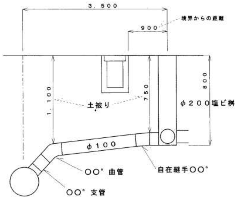
( 縦 断 図 )
