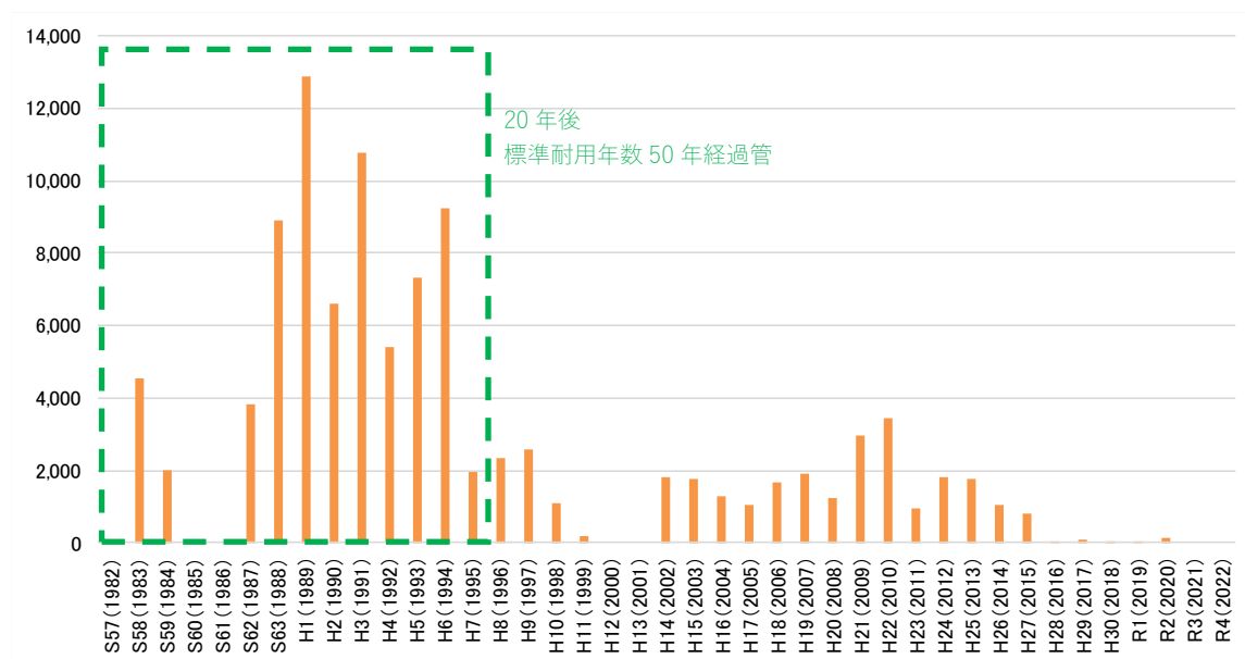
図 3-2 污水管きょ延長【単年度】（特定環境保全公共下水道）
