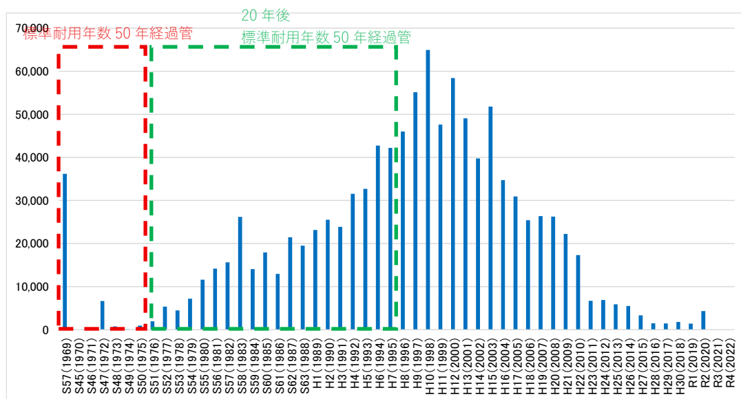
図 3-1 污水管きょ延長【単年度】（流域関連公共下水道）
