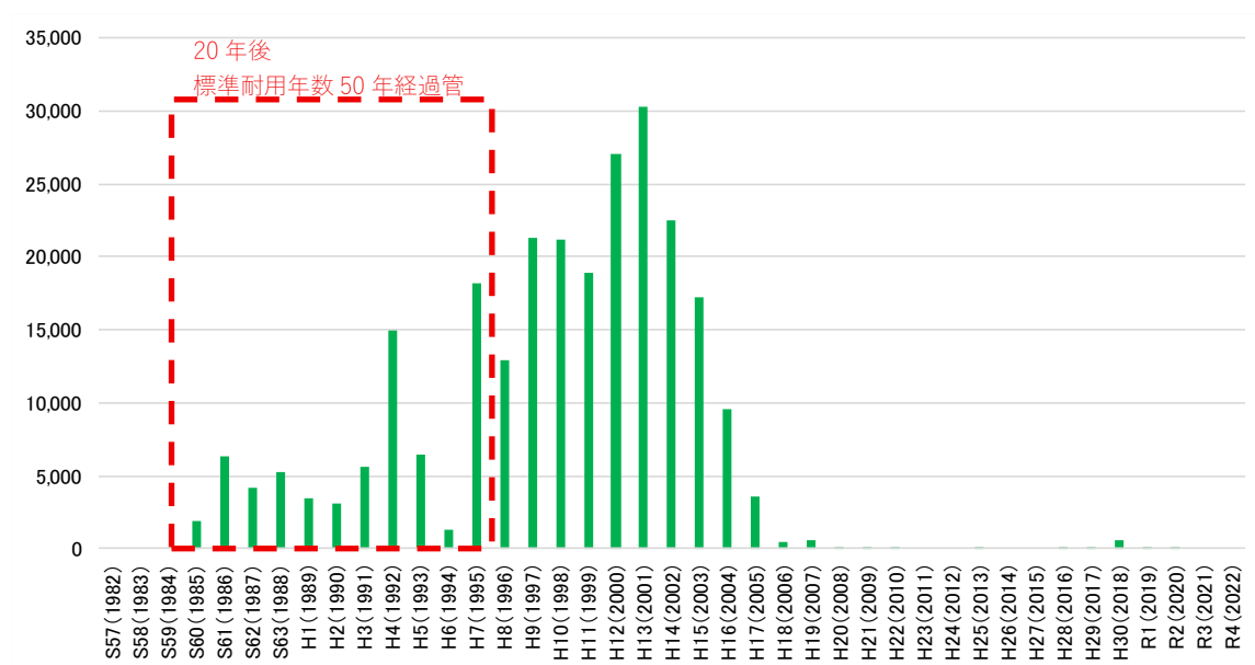
図 3-3 汚水管きょ延長【単年度】（農業集落排水処理事業）
