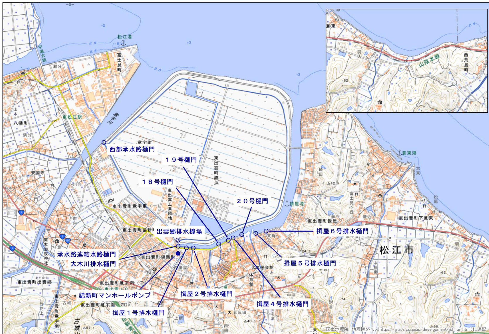
図 1-1 雨水施設 位置図 (4/4)
